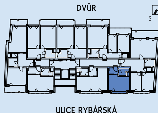
PŮDORYS 4.NP
